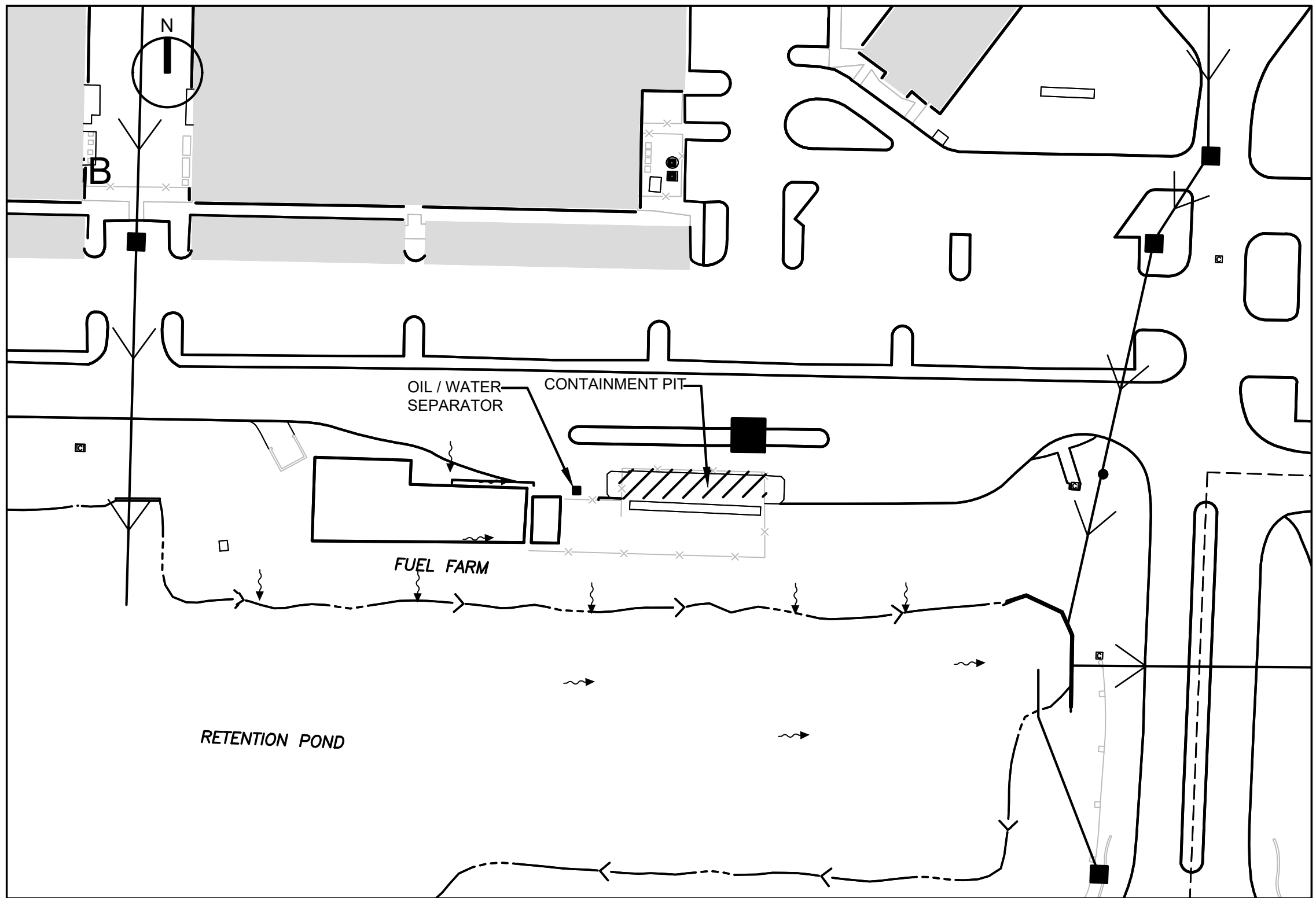
DETAIL "C" SCALE: 1" = 50'
